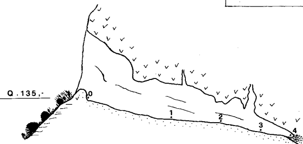
SEZ. LONGIT.
